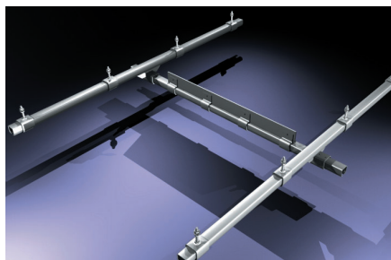
Systemy lekkich suwnic i żurawi
