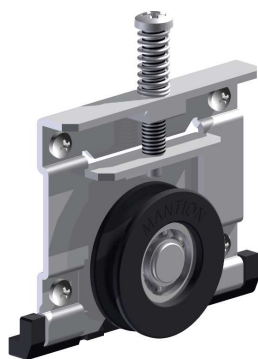
215-215 wózek dolny
